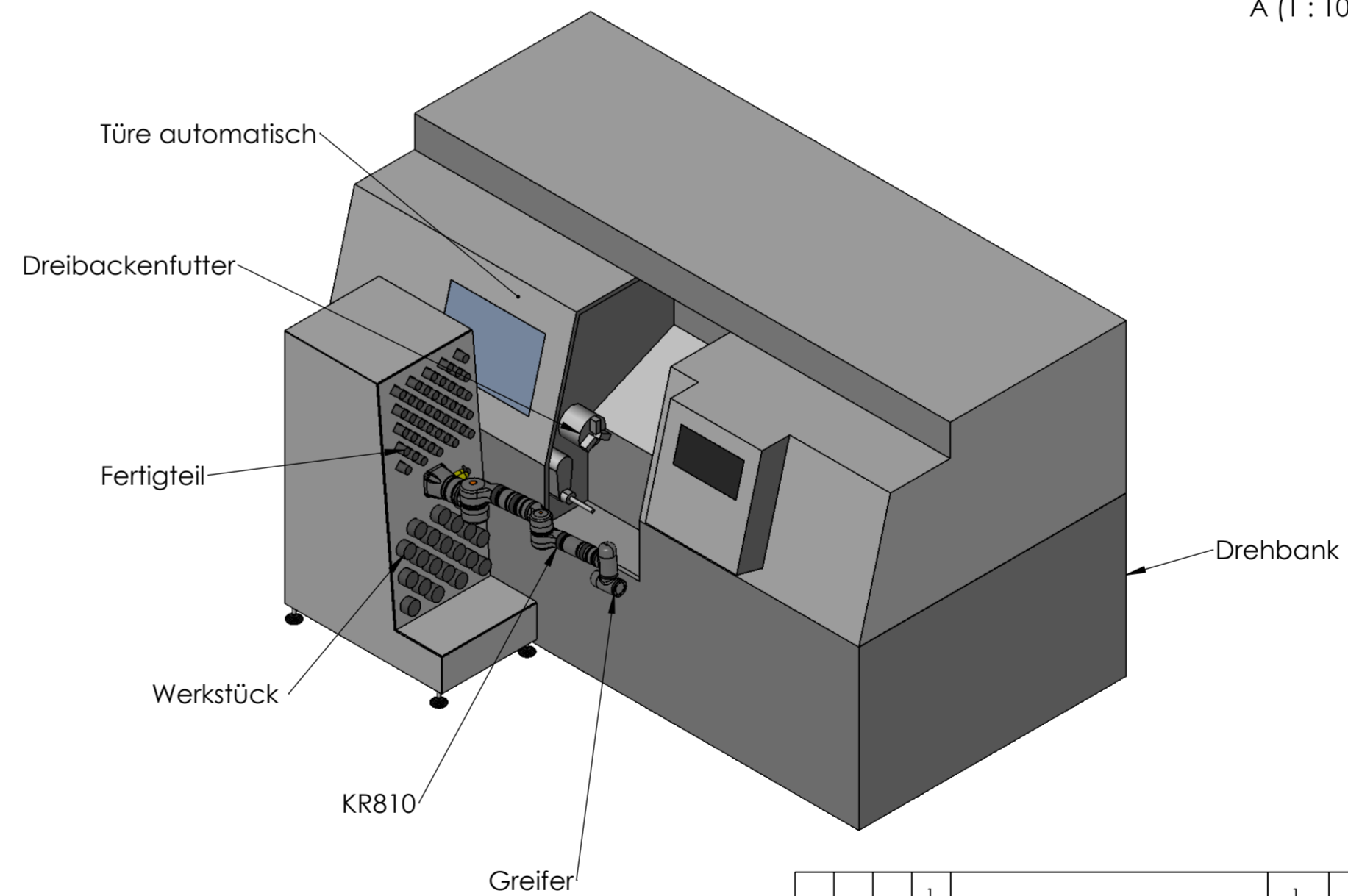
A (1 : 10)
